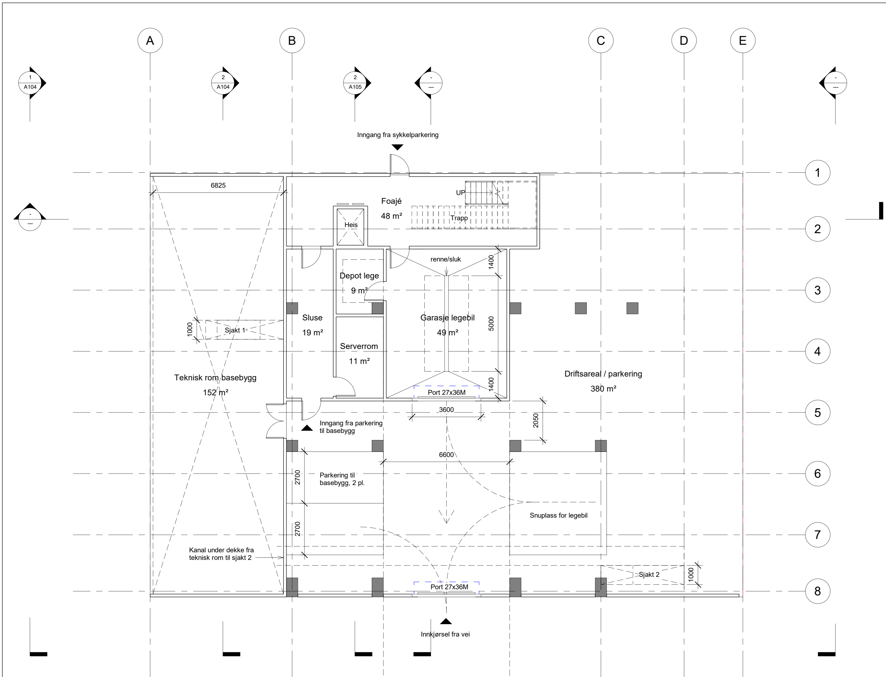
1 Plan 01 rotert 1 : 100
